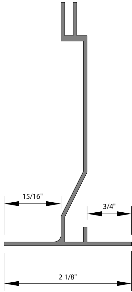
T-MULLION
